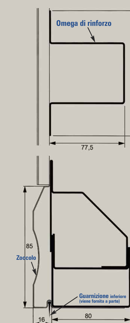
Particolare guarnizione antiscivolo in base alla direttiva macchine UNI-EN.
