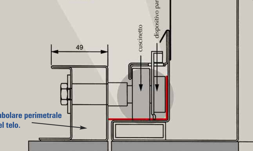
Particolare paracadute di emergenza.
