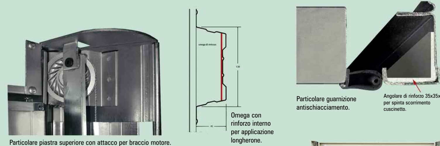
Particolare piastra superiore con attacco per braccio motore.
